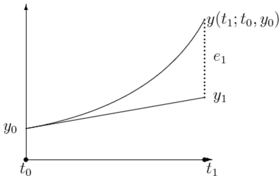
Figure 2.1: El método de Euler. El error e_1 es |y_1 - y(t_1; t_0, y_0)| .
